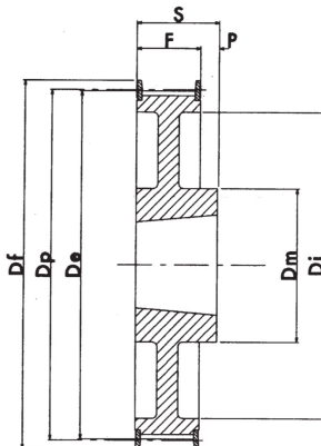
esecuzione 6F
