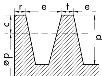
Gole lavorate secondo norma ISO 4183
