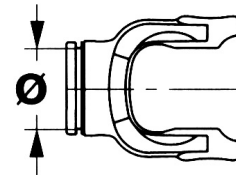
FORCELLA PER TUBO INTERNO
