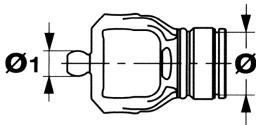
FORCELLA PER TUBO ESTERNO
