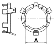
Anello di supporto tipo "100"
