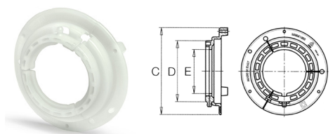
Anello di supporto tipo "Global"
