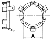
Anello di supporto tipo "100"
