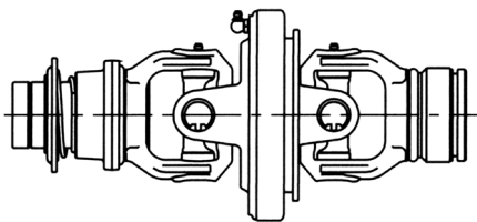
GIUNTO COMPLETO PER TUBO ESTERNO
