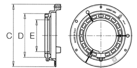
Anello di supporto tipo "Global"
