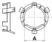
Anello di supporto tipo "100"
