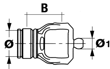
FORCELLA PER TUBO INTERNO
